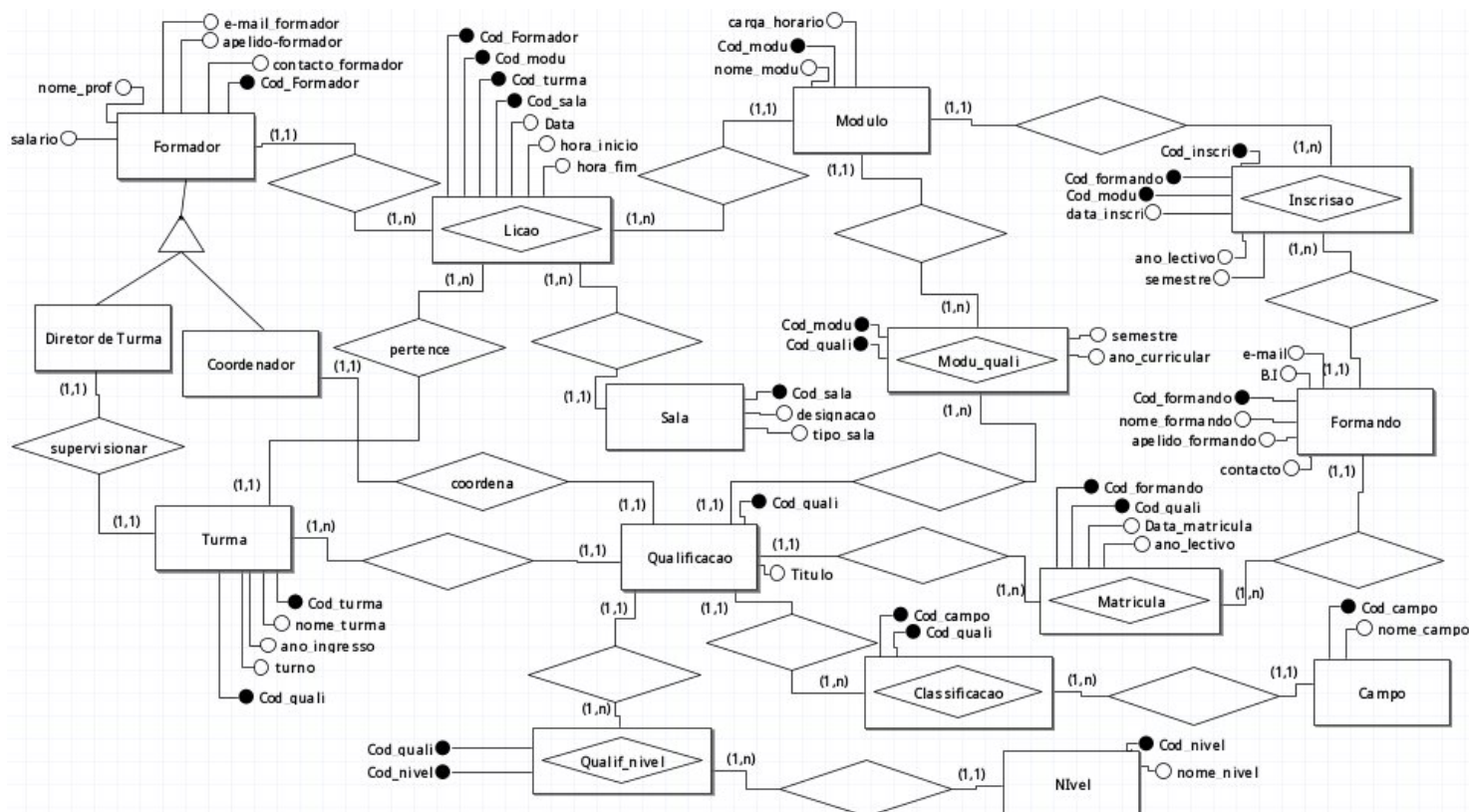
Figura 2 : diagrama entidade relacionamento refinado
