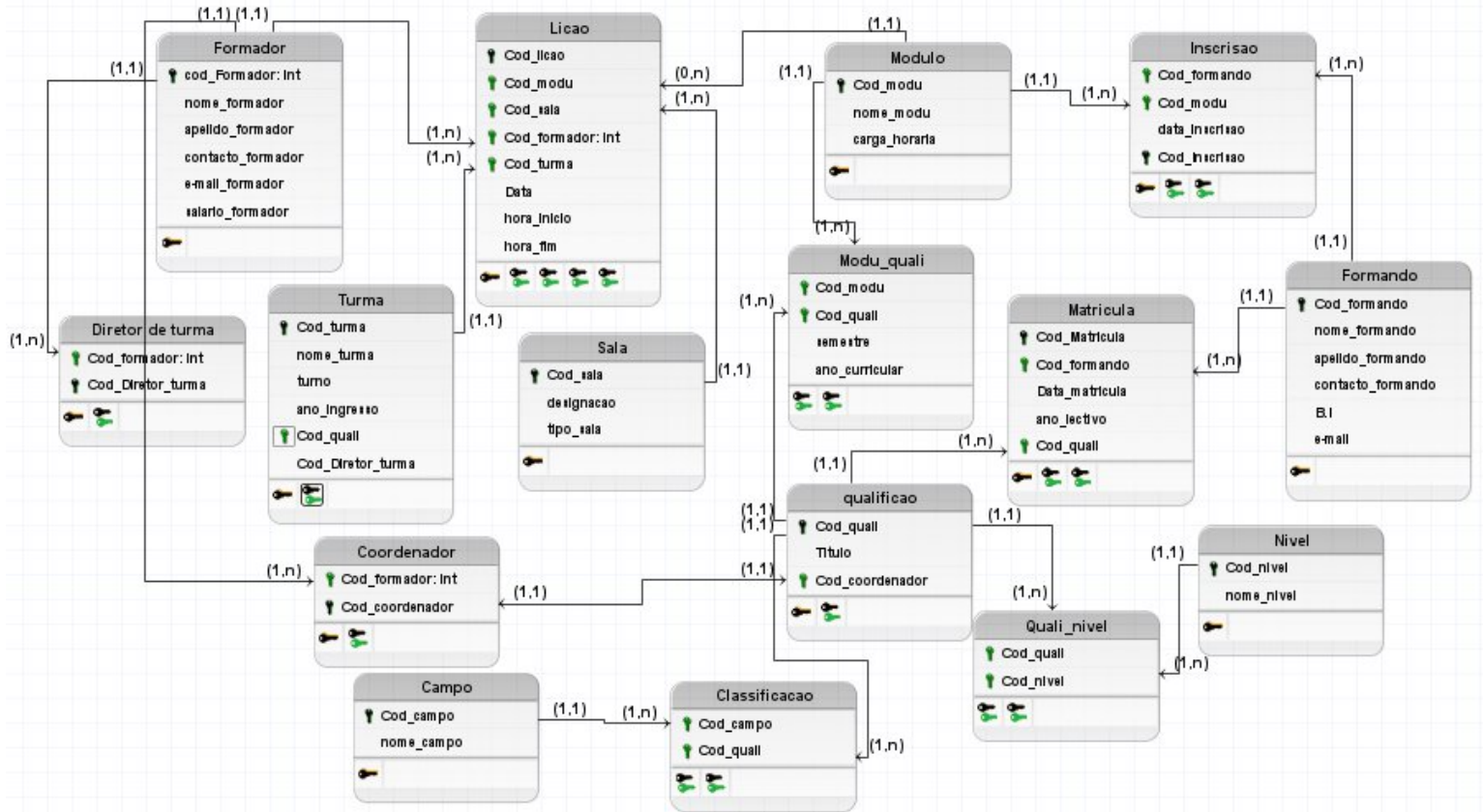
Figura 3: Modelo lógico de entidades
