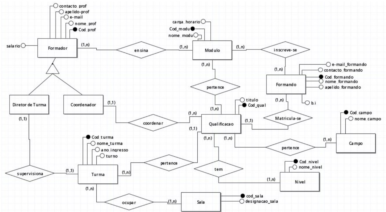
Figura1: diagrama de entidade relacionamento normal
