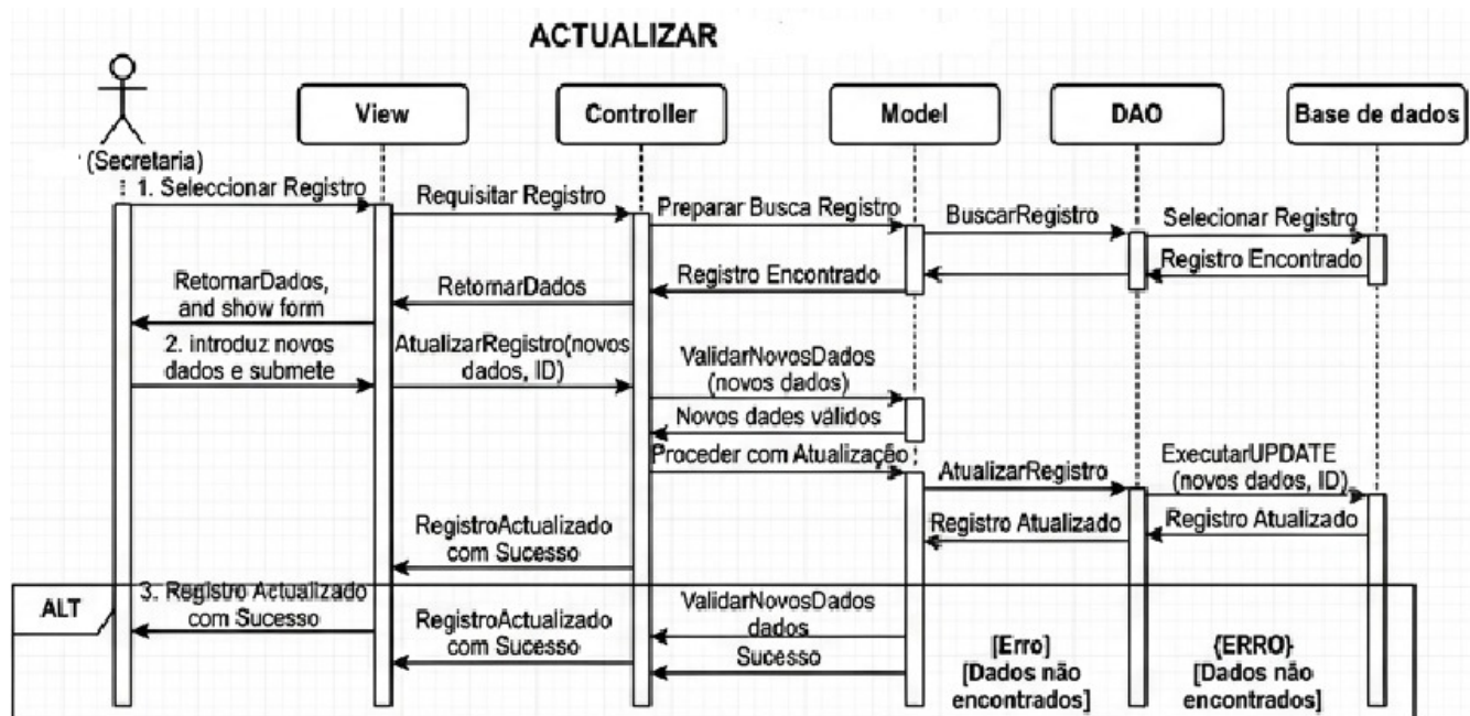
Figura 24: Diagrama de sequencia de atualização de objeto
