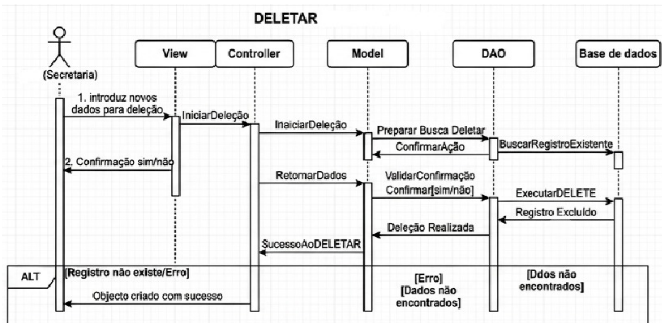
Figura 25: Diagrama de sequencia de remoção de objeto
