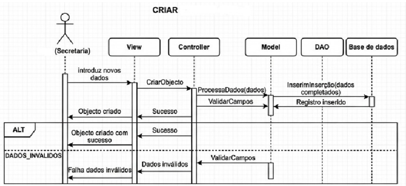
Figura 22: Diagrama de sequencia de Inserção de objeto
