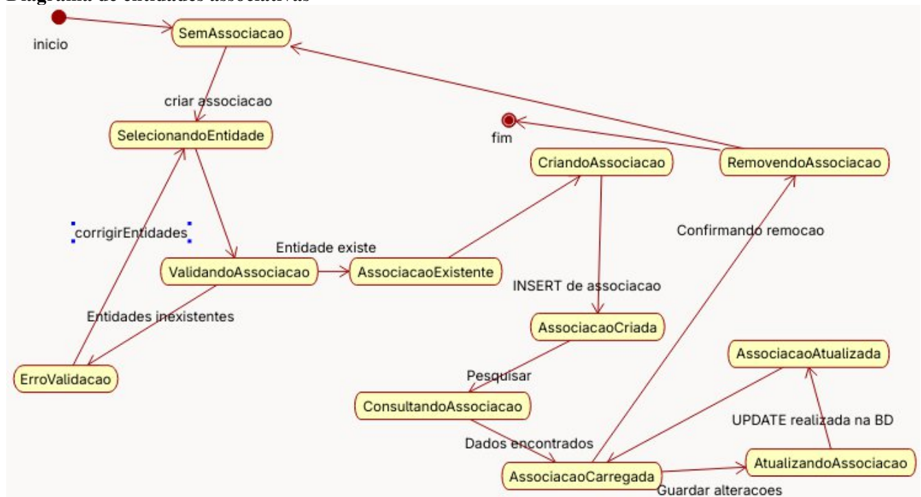
Figura 27: diagrama de estados de entidades associativas
