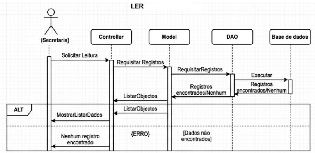
Figura 23 Diagrama de sequencia de consulta de objeto
