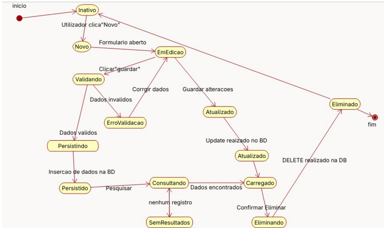
Figura 26: diagrama de estado genérico
